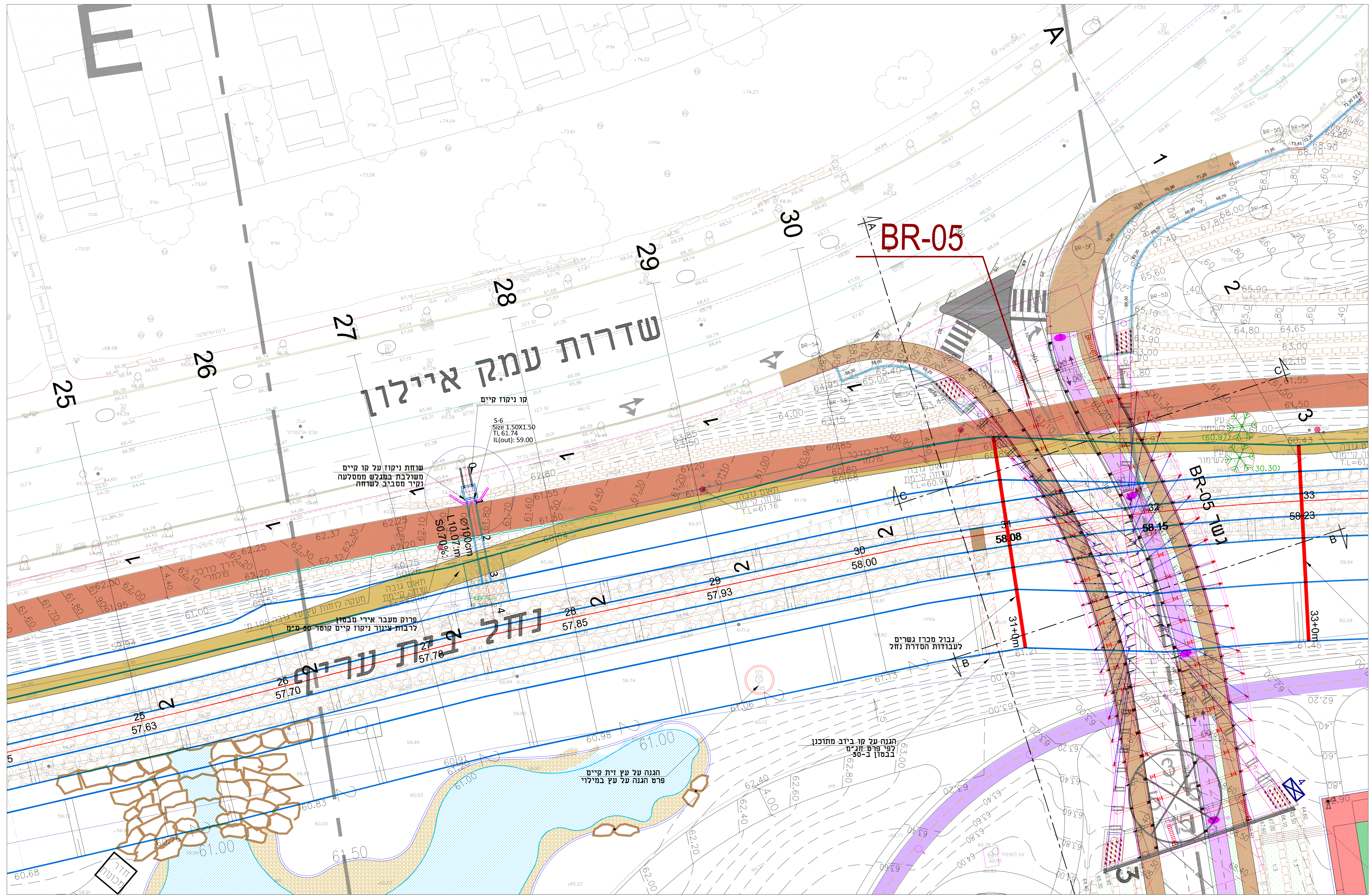
תכנית גשר BR-5 קנ"מ: 1:200
